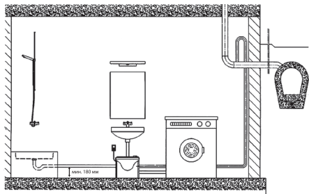
3-сур. Liftaway C қондырғысын құрастыру үлгісі
